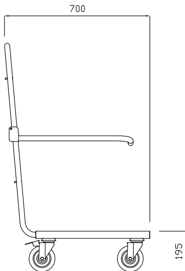
Boven aanzicht
